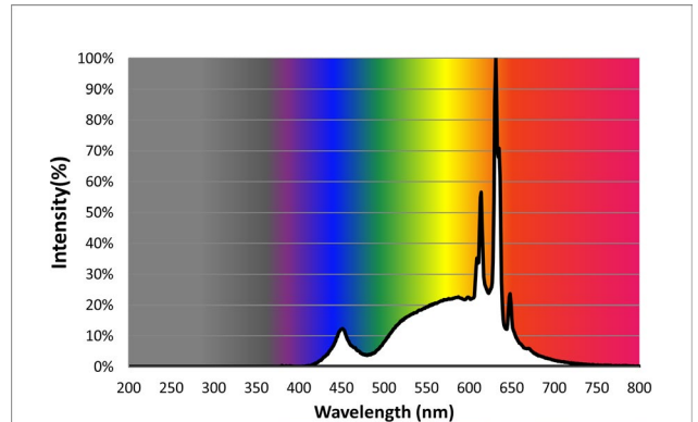
WiZ Pro A60 B22 RGBTW 8W 230V
